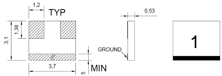
FAC0601 2W( Al_2O_3 )
