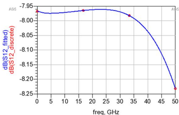
裸片在探针台的测试结果
