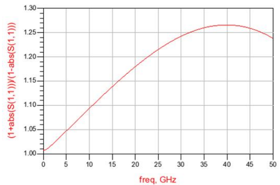
加 300um 双键合线的测试结果
