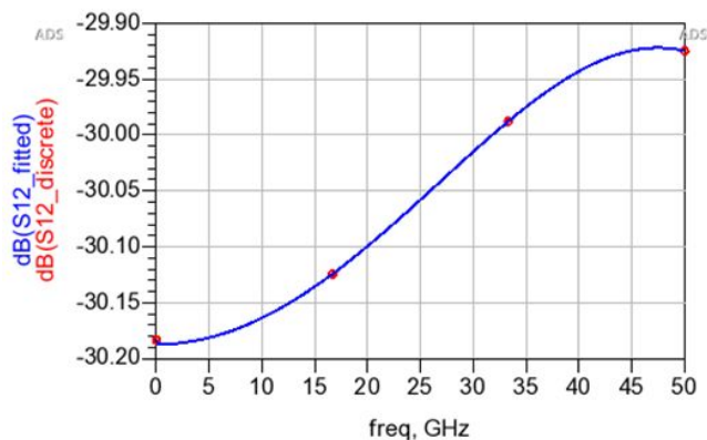
裸片在探针台的测试结果
