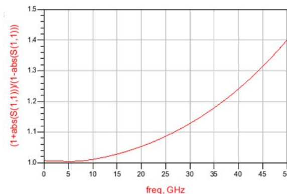
裸片在探针台的测试结果
